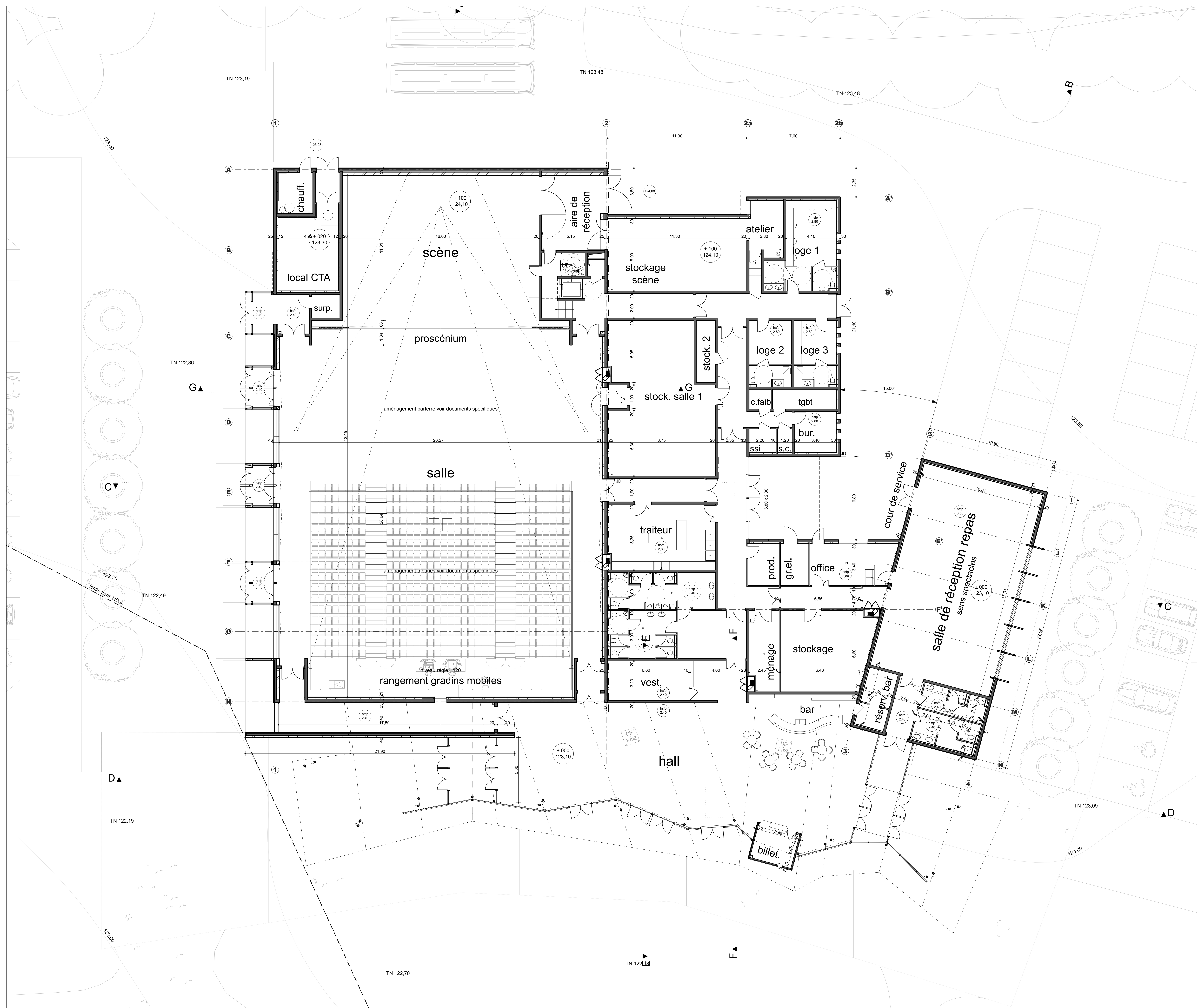
PLAN NIVEAU INTERMÉDIAIRE
